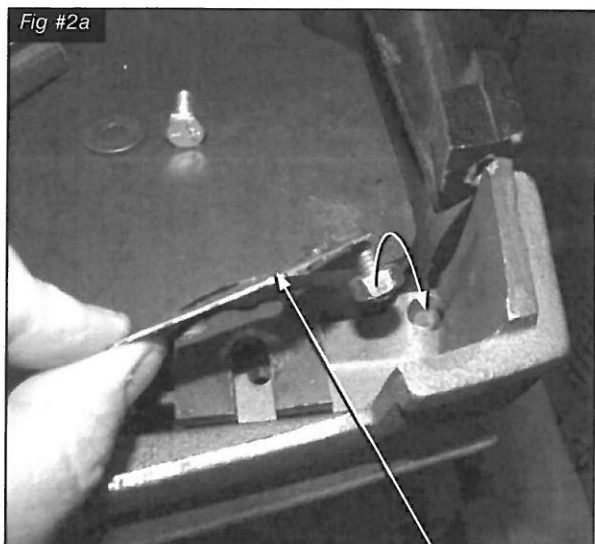
DOOR PIN RETAINER
